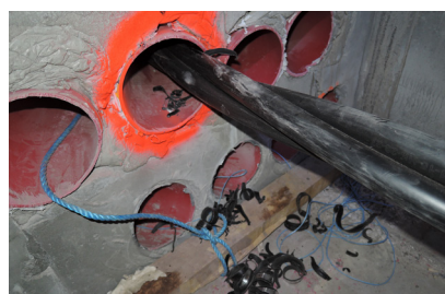
Eksempel på skadet kabel ved ikke bruk av trompetending.
