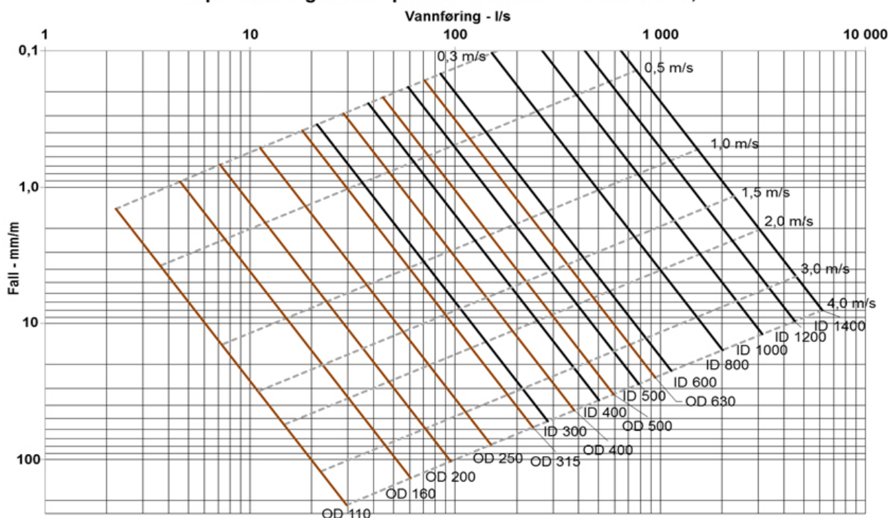
Kapasitetsdiagram for plastrør med bruksruhetsverdi 0,25
