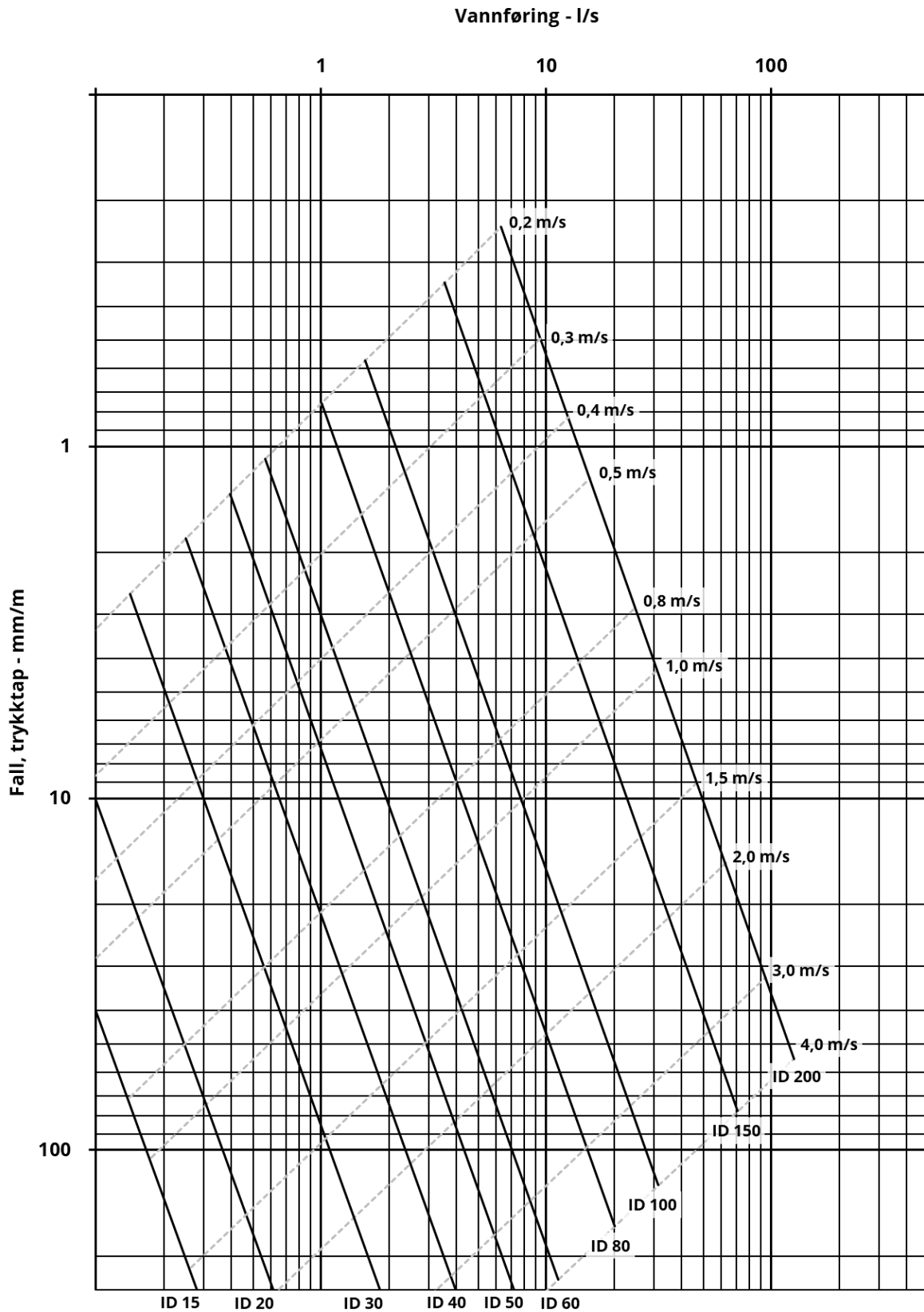
Vannføringsdiagram for rør med innvendig diameter fra 15 mm til 200 mm ved 10^{\circ}\text{C} . k = 0,01\text{ mm}
